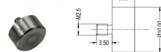
平头 (φ10mm) flat head (φ10mm)
