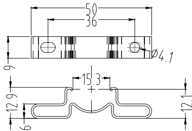
标配：五金支架
