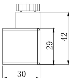
KTF: 赫斯曼插头式 (标配)
