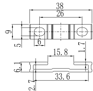
可选铝合金支架 Optional aluminum bracket
