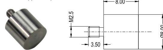
平头 (φ8mm) flat head (φ8mm)
