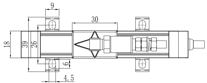
安装支架 Mounting bracket
