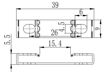
标配五金支架
