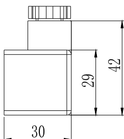
KTC11/KTC1/LWH: 标准赫斯曼插头式 Standard Hersman plug type
