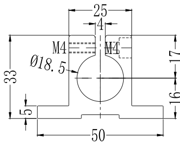
可选：铝合金支架
