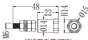
标准万向节(可选)
