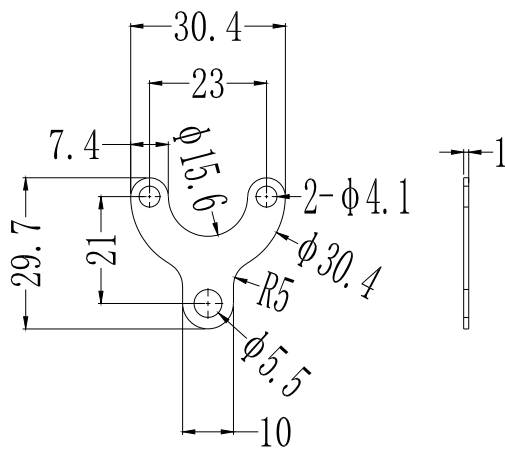
磁环安装导片
