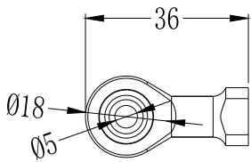
可选：鱼眼接头
