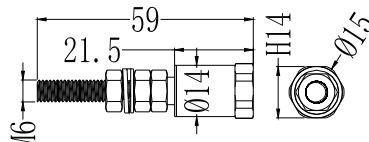
加长万向节(可选)
