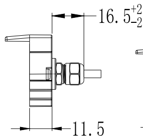
KTFC: 防水接头式
