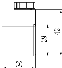
KTC11S: 标准赫斯曼插头式 Standard Hersman plug type
