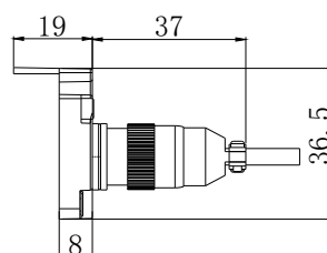
KTF1P: 航空插头式 Aviation plug type
