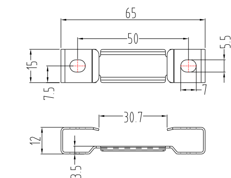
安装支架 installing support
