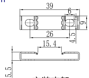
安装支架 Mounting bracket
