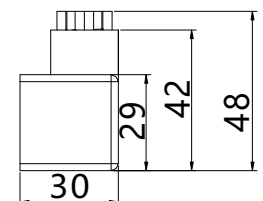
H4赫斯曼小插头 H4 Hesmann small plug
