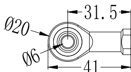
鱼眼接头(默认)
