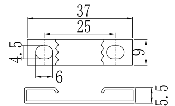
安装支架 Mounting bracket
