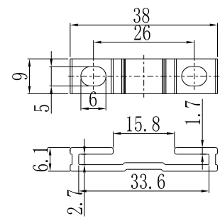
可选铝合金支架 Optional aluminum alloy bracket
