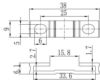
可选铝合金支架
