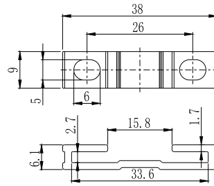
可选铝合金支架 Optional aluminum bracket
