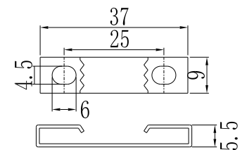
安装支架 Mounting bracket
