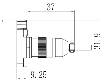
KTC11P/KTC1P/LWHP: 航空插头式 Aviation plug
