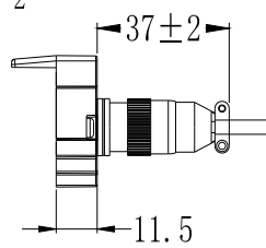
KTFP: 航空插头式
