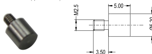
平头 (φ5.2mm) flat head (φ5.2mm)
