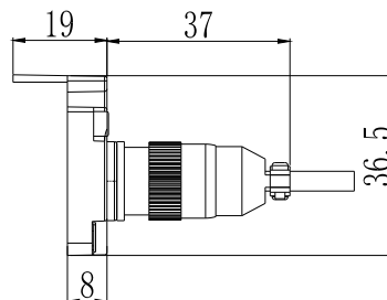
KTC11SP: 航空插头式 Aviation plug
