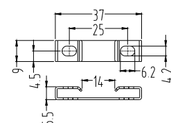
安装支架 Mounting bracket
