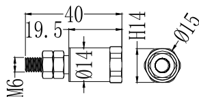
缩短万向节(可选)
